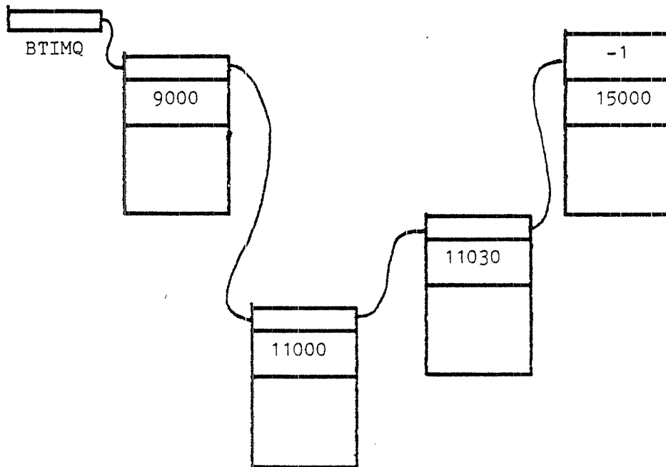
Fig. 13. Time queue
